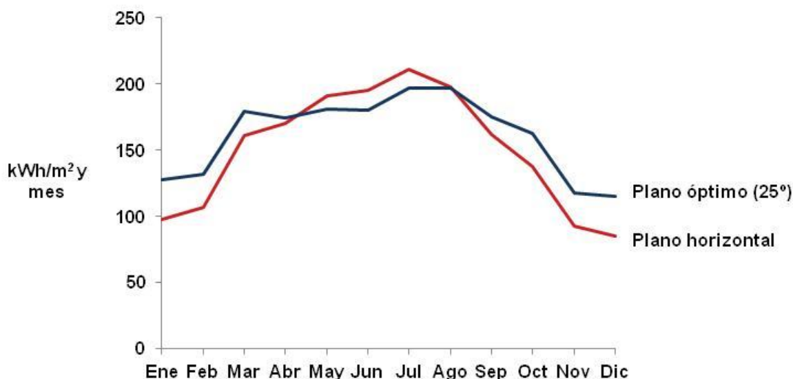
Ilustración 12: Irradiación global media por m 2 en San Andrés y Sauces para estructura fija
